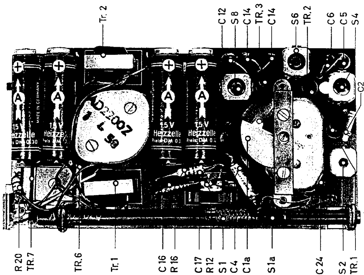
Empfänger - Chassis, Rückansicht
