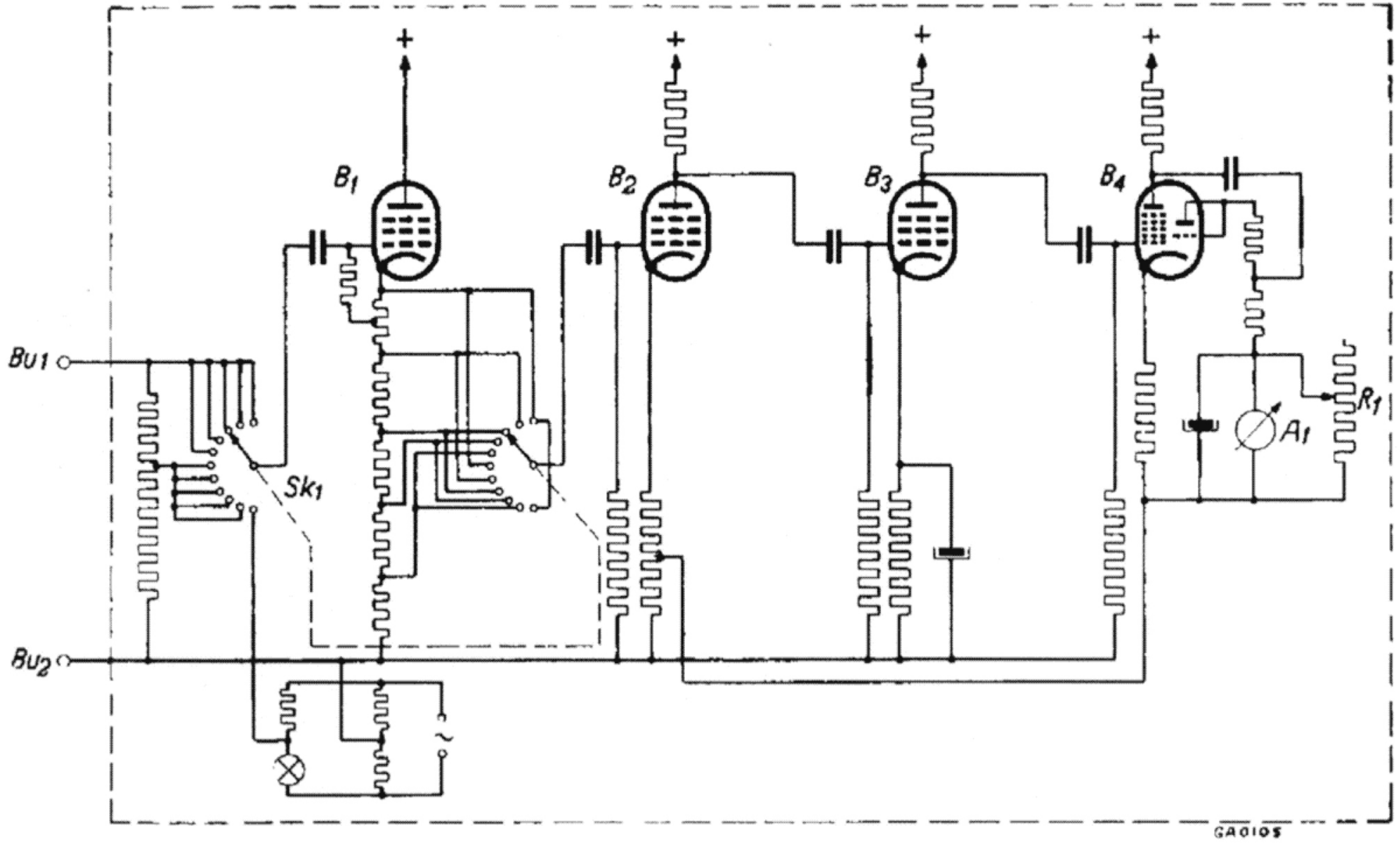
Fig. 1 Vereenvoudigd principeschema
