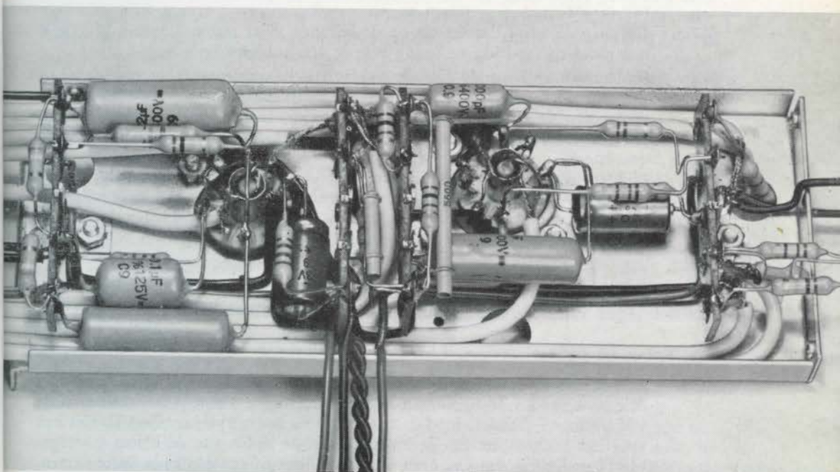
Afb. 2. De gemonteerde stuurversterker (kleine montageplaat).
