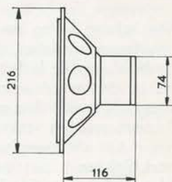
Afb. 10. Afmetingen in mm van de luidsprekers 9710...
