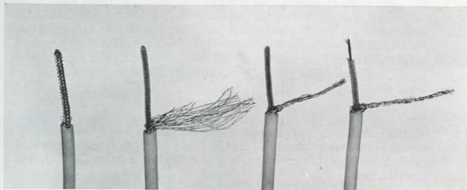
Afb. 1. Het gereedmaken van een stukje afgeschermd snoer in vier fazen.
